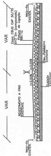
CORTE B-B - CBUQ SEM ESCALA
